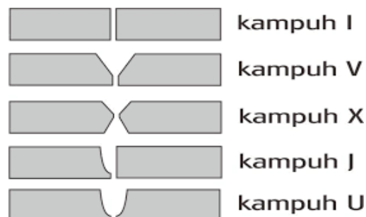
Gambar 2.14 Jenis-Jenis Kampuh
