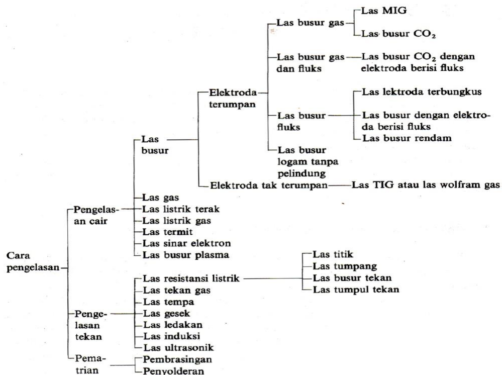
Gambar 2.1 Klasifikasi Cara Pengelasan
