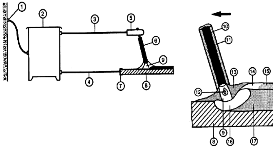
Gambar 2.4 Las Listrik
