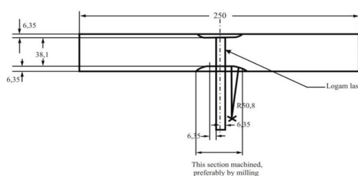
Gambar 2.17 Batang Uji Tarik
