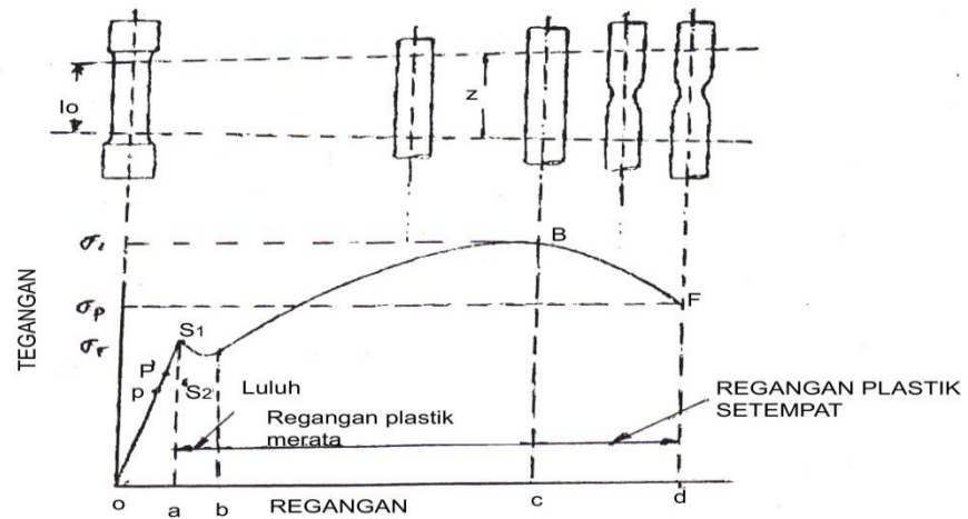
Gambar 2.18 Kurva tegangan – regangan
