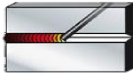
Gambar 2.6 Posisi 2G
