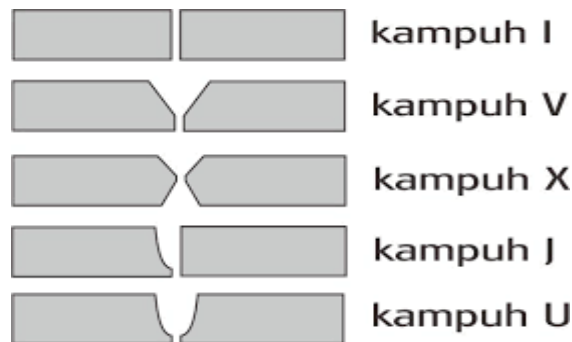
Gambar 02.14 Jenis-Jenis Kampuh
