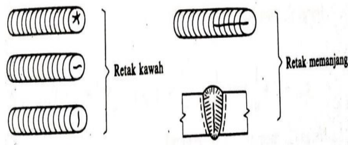
Gambar 2.11 Retak Panas
