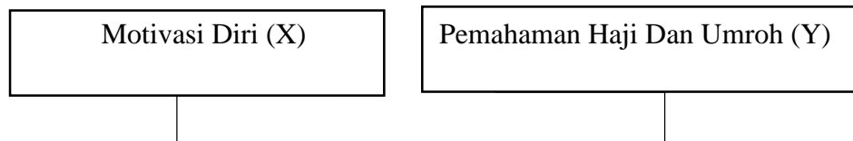
Gambar II.1 Kerangka Berpikir
