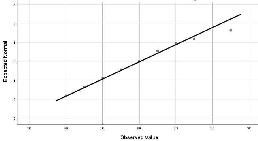
Normal Q-Q Plot of Posttest Kelas eksperimen
