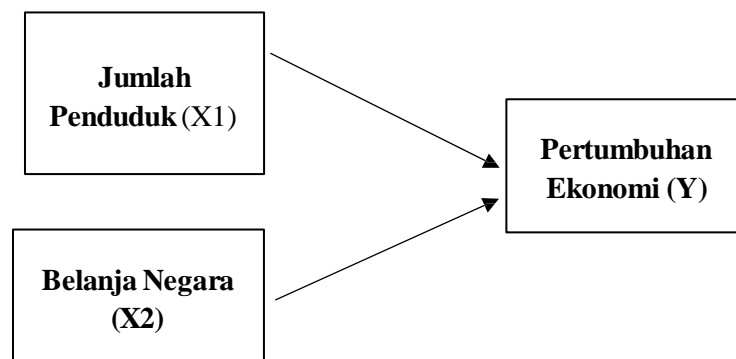
Gambar 2.2 Kerangka Konseptual
