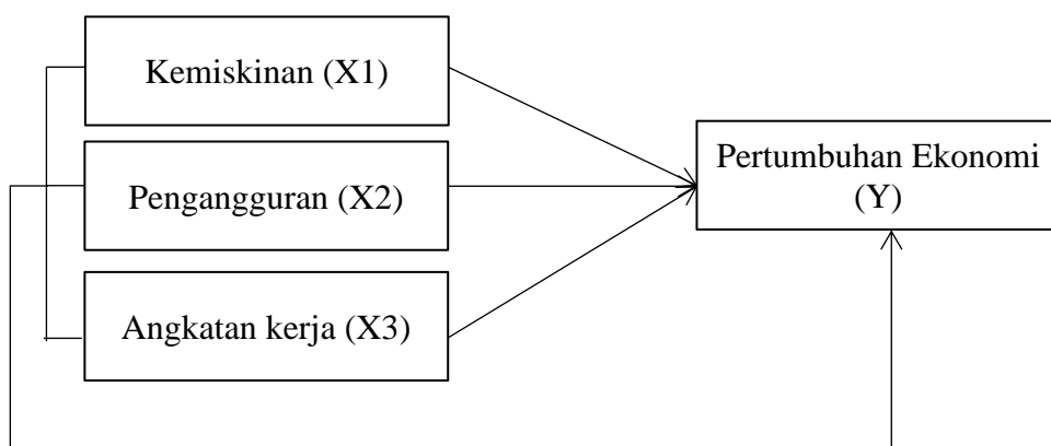
Gambar II.1. Kerangka Konseptual
